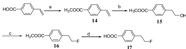
Scheme 2. Reagents: (a) (CH 3 ) 3 OBf 4 , CH 2 Cl 2 , N(C 2 H 5 ) 3 ; (b) (1) BH 3 /THF, (2) NaOH, 35% H 2 O 2 ; (c) (C 2 H 5 ) 2 NSF 3 , CH 2 Cl 2 ; (d) (1) NaOH, CH 3 OH/H 2 O, (2) HCl.
