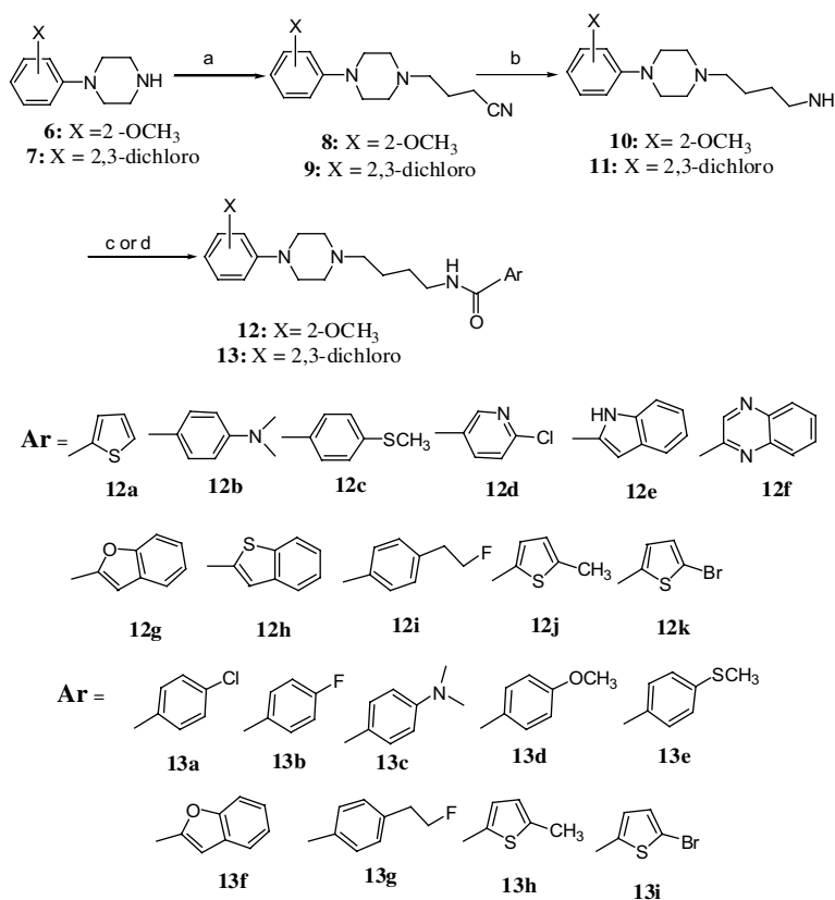
Scheme 1. Reagents: (a) 4-bromobutyronitrile, N(C 2 H 5 ) 3 , CH 2 Cl 2 ; (b) LiAlH 4 , THF; (c) (1) ArCOOH, ClCOOC 2 H 5 , N(C 2 H 5 ) 3 , (2) 10 or 11 ; (d) ArCOOH, 10 or 11 , Bop-Cl, (C 2 H 5 ) 3 .
